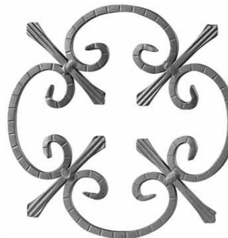
Diametro mm. 250 ART. PAN12L Quadro mm. 8 Tachettato
